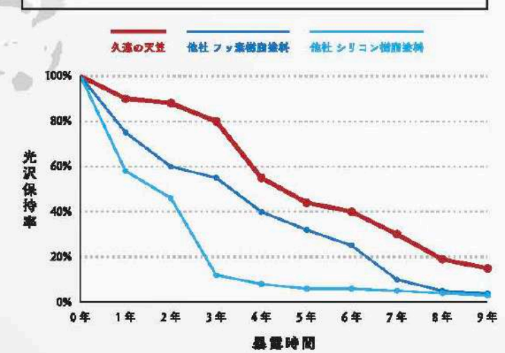
宮古島暴風試験における促進耐候比較
